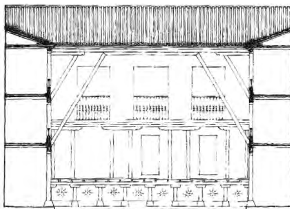
SECCION TRANSVERSAL
